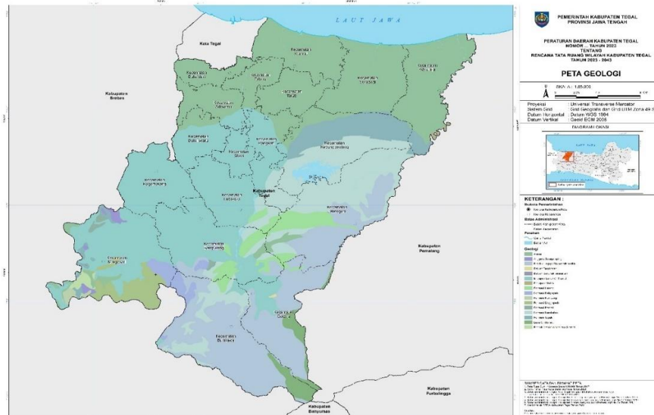
Gambar 2. 4 Peta Geologi Kabupaten Tegal
