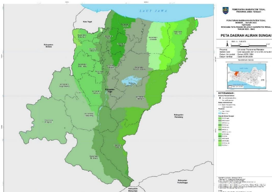
Gambar 2. 5 Peta Daerah Aliran Sungai
