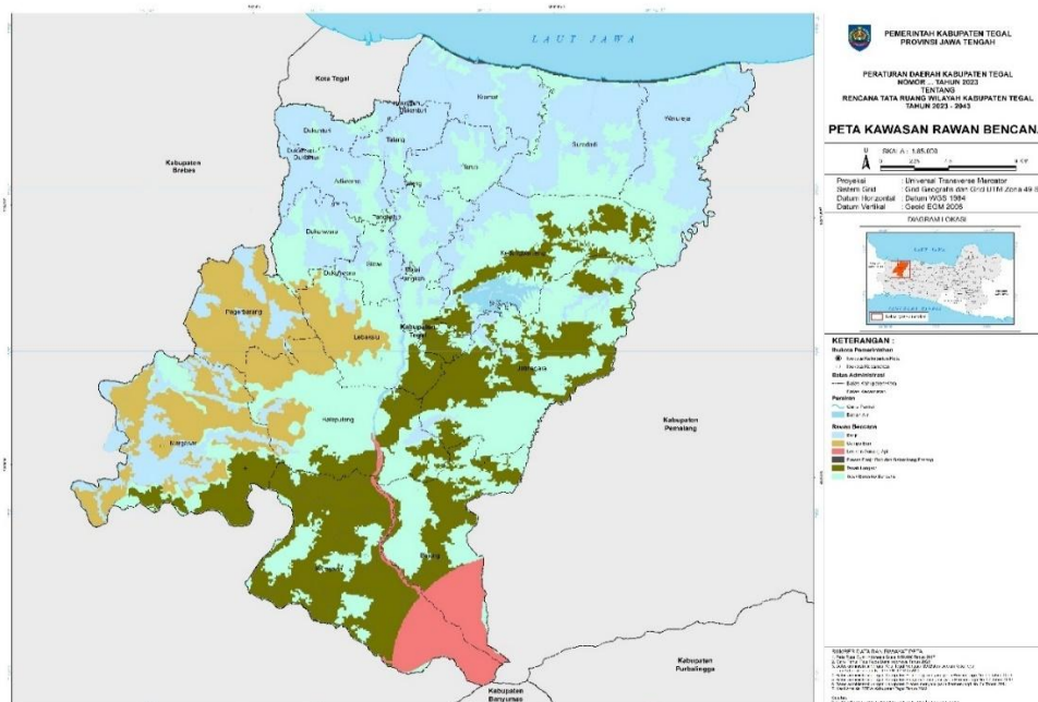
Gambar 2. 7 Peta Kawasan Bencana Alam
